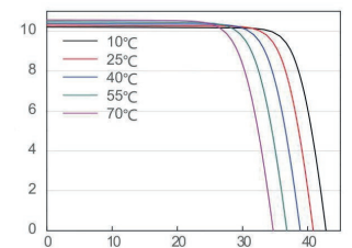
Wykres prąd-napięcie: (A-HCM320M)
